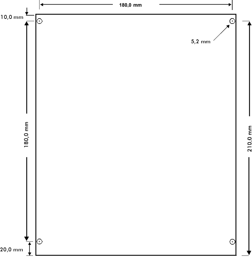
Afbeelding 4. Boorafmeting
